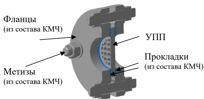
Внешний вид УПП с комплектом монтажных частей (показано в разрезе)
